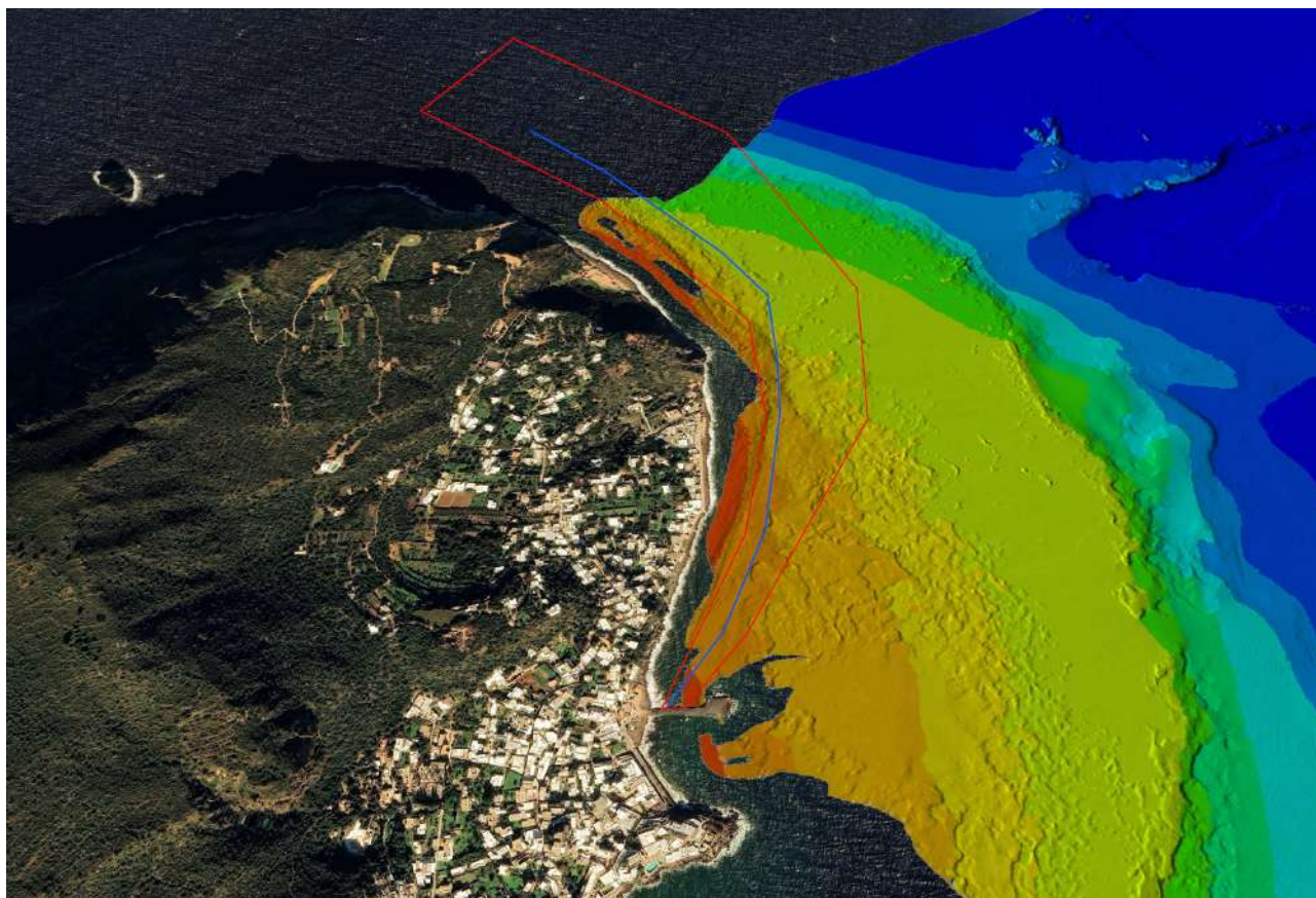
Figura 1 – Percorso ideale del cavo (in blu) con un tracciato che resterà comunque confinato all'interno del poligono in rosso
